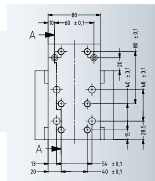
ER-108194 RCS5 Pinza con gancio di carico
